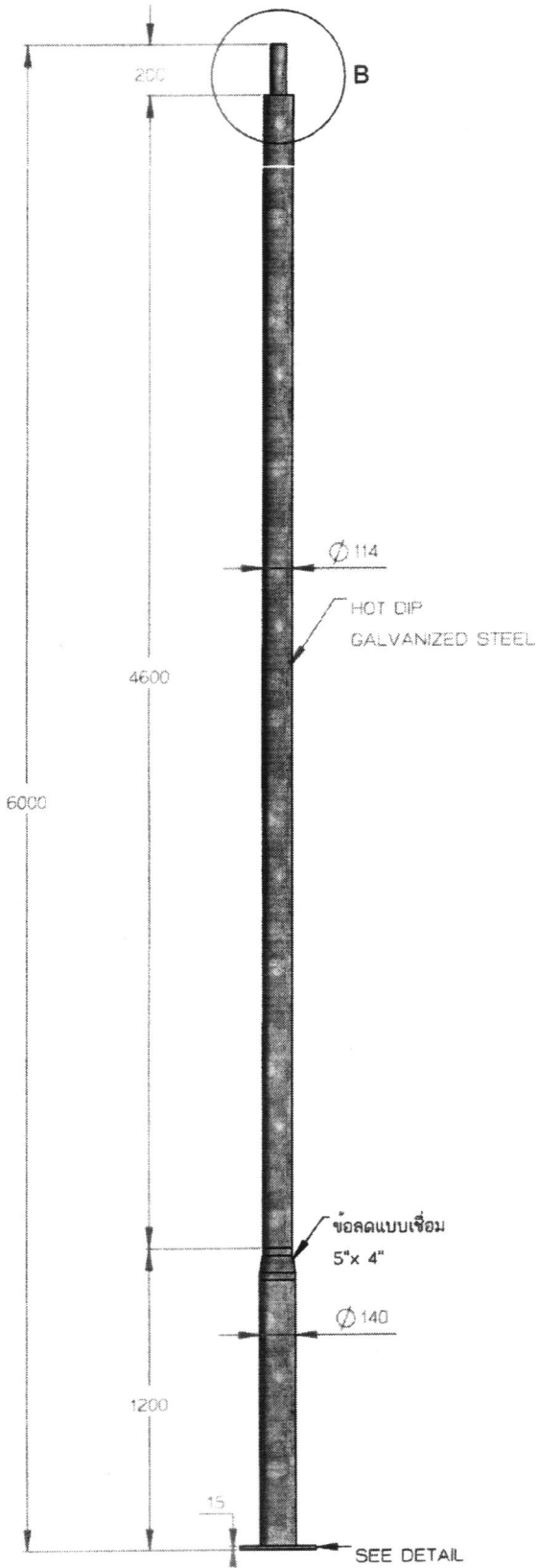
HI-WCS-060:เสาทอมสูง6เมตรขนาด5นิ้วด4นิ้ว SCALE 1 : 28
